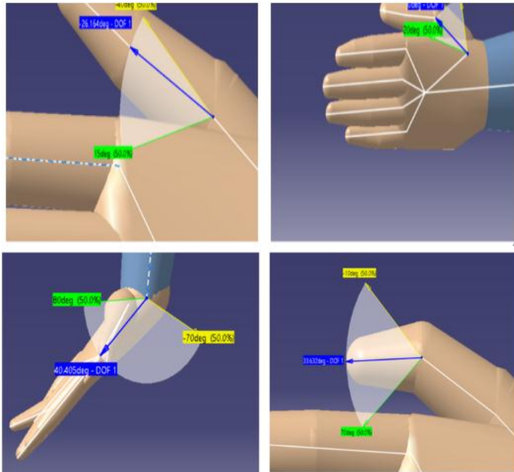
شکل ۳- درجه آزادی انگشت شست دست و میج دست
